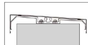
内勾配笠木(見付60mm)
